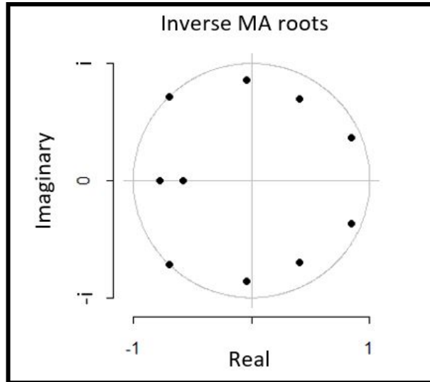
Figura 6. Prueba de estabilidad del ARIMA (0,1,10)
