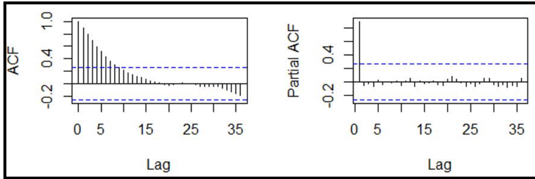
Figura 3. Gráficos de ACF y PACF para el modelo en fase de entrenamiento.
