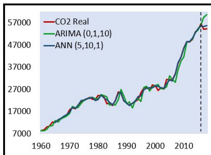
Figura 7. Rendimiento de predicción del mejor modelo ARIMA (0,1,10) y el mejor modelo de red neuronal Feed Forward ANN(5,10,1) para conjuntos de entrenamiento (1960-2014) y de prueba (2015-2018) de las emisiones de CO 2 en Perú actualizado por el Banco Mundial al 2021.
