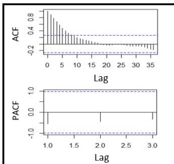
Figura 2. Gráficos de los correlogramas (ACF y PACF) para el modelo en fase de entrenamiento.
