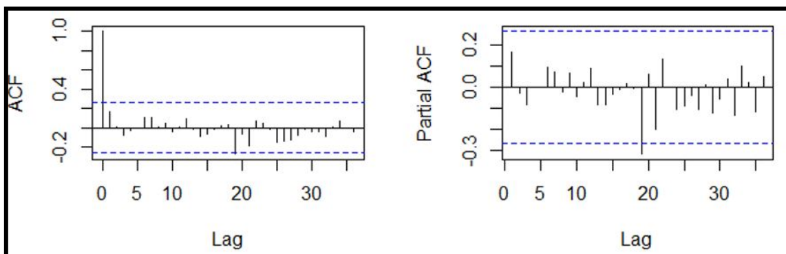
Figura 5. Gráficos de ACF y PACF para la serie [[CO]]_2^\lambda en fase de entrenamiento. Y por la prueba de Dick Fuller tenemos un p\text{-value} = 0.0402 < 0.05 la cual nos dice según la H_0 que ya es estacionario y a partir de ello podemos identificar a nuestros modelos, las cuales en resumen son: ARIMA(1,1,8), ARIMA(1,1,7), ARIMA(1,1,6), ARIMA(7,1,1)
