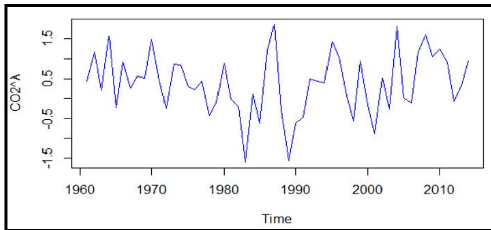
Figura 4. Gráfico de la serie [[CO]]_2^\lambda diferenciada con d = 1 .
